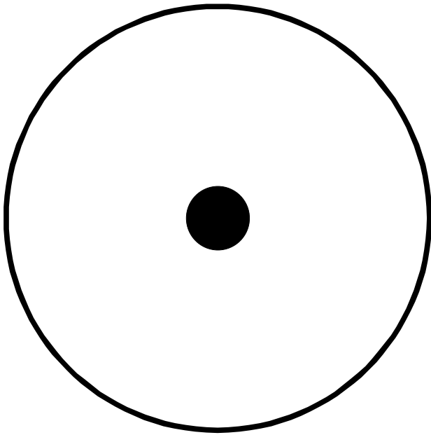
水素
