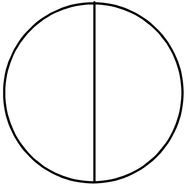
窒素
