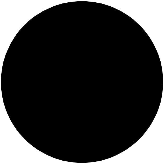
炭素
