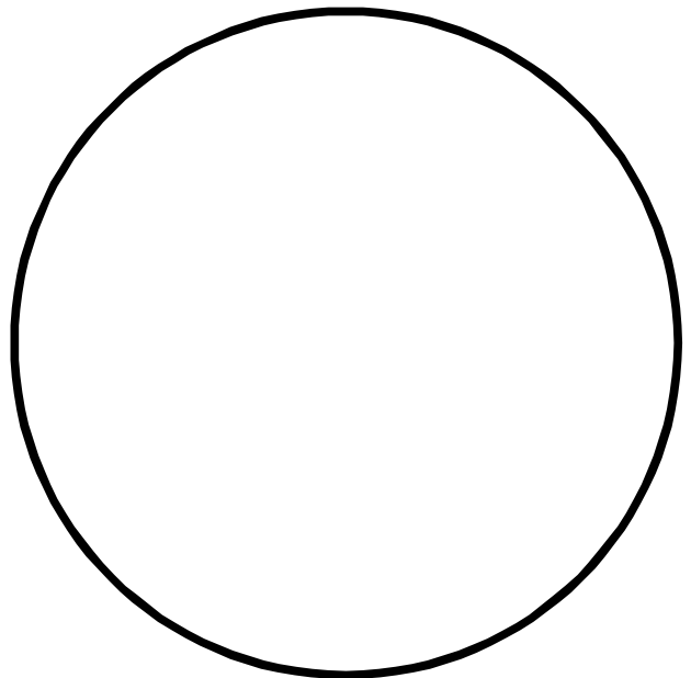
酸素
